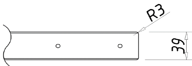
Планка стыковочная угловая R3
