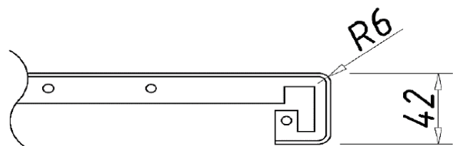
Планка стыковочная прямая U-закругление R6
